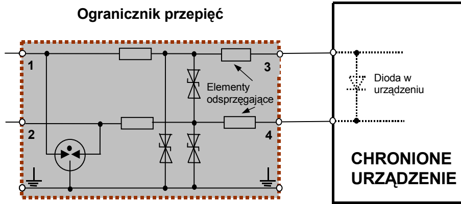
Rys.10. Dodatkowe elementy odsprzęgające w układzie chroniącym przed przepięciami
