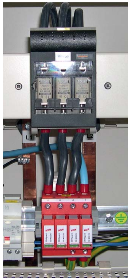
Rys. 2. Przykład dobezpieczenia ogranicznika przepięć typu 2 w rozdzielni
