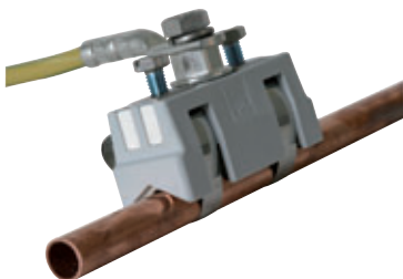
Ex-BRS 27 Art.-Nr. 540 821 Klemmbereich \varnothing 6 mm - 3/4"
