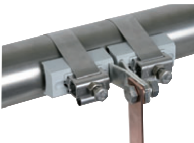
Ex-BRS 90 Art.-Nr. 540 801 Klemmbereich \varnothing 3/4" - 3" Ex-BRS 300 Art.-Nr. 540 803 Klemmbereich \varnothing 3" - 300 mm
