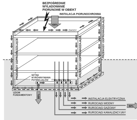
Rys.1. Przykładowy rozptyw prądu piorunowego w obiekcie budowlanym
